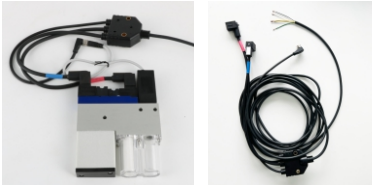
MCP(20至30)-RD 控制线连接示意图 集成线 (开关线+电磁阀线)
